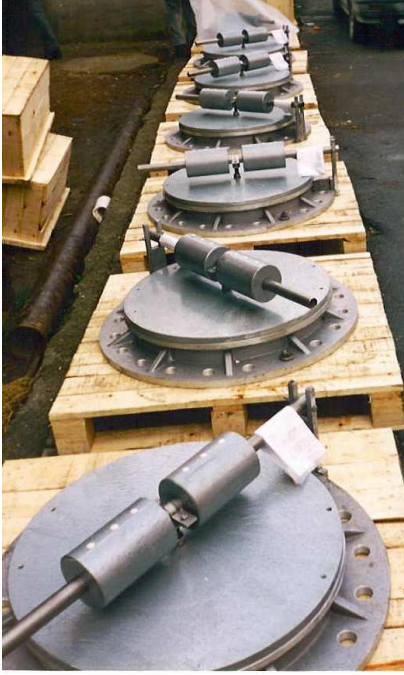
Emergency Vents Acil Dışatım Ventilleri
